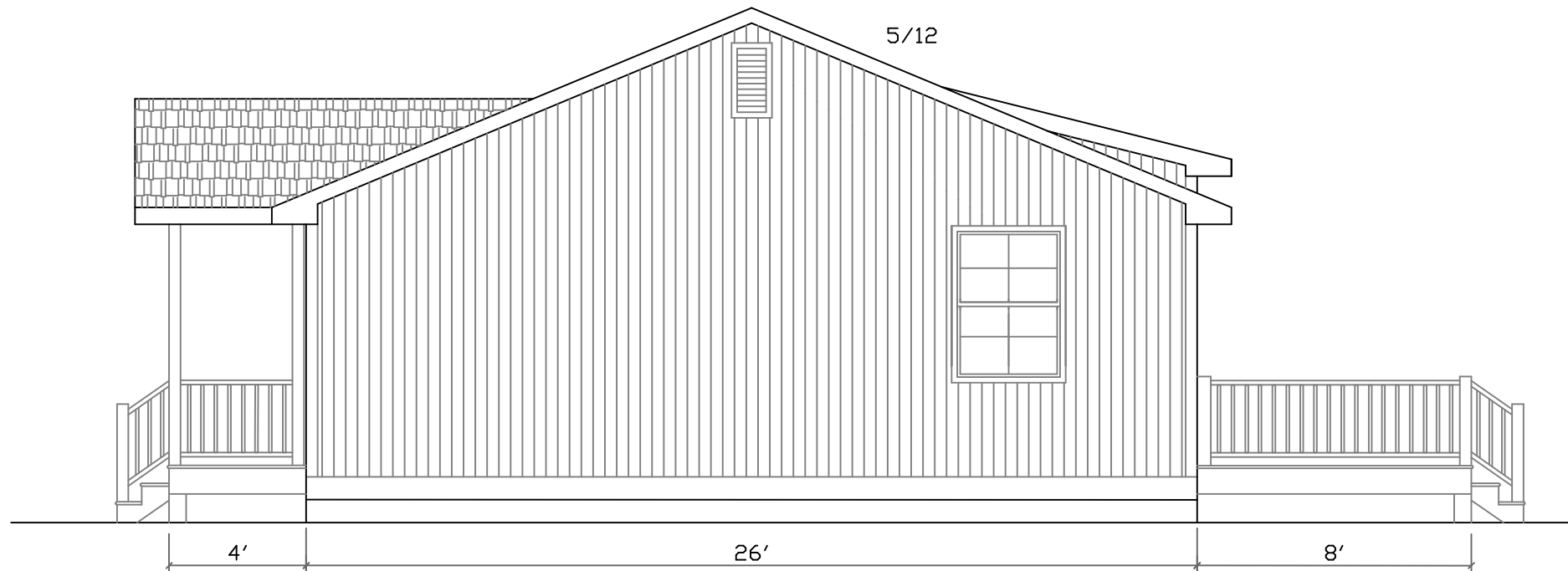
RIGHT ELEVATION
